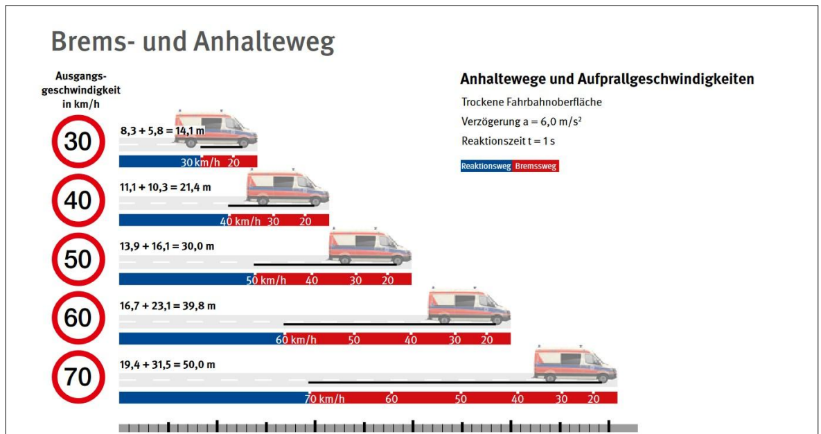
Abbildung 18: Brems- und Anhalteweg bei unterschiedlichen Geschwindigkeiten
